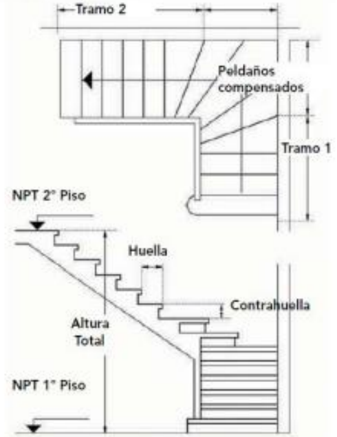
Escalera de dos tramos en ángulo recto con peldaños compensados
